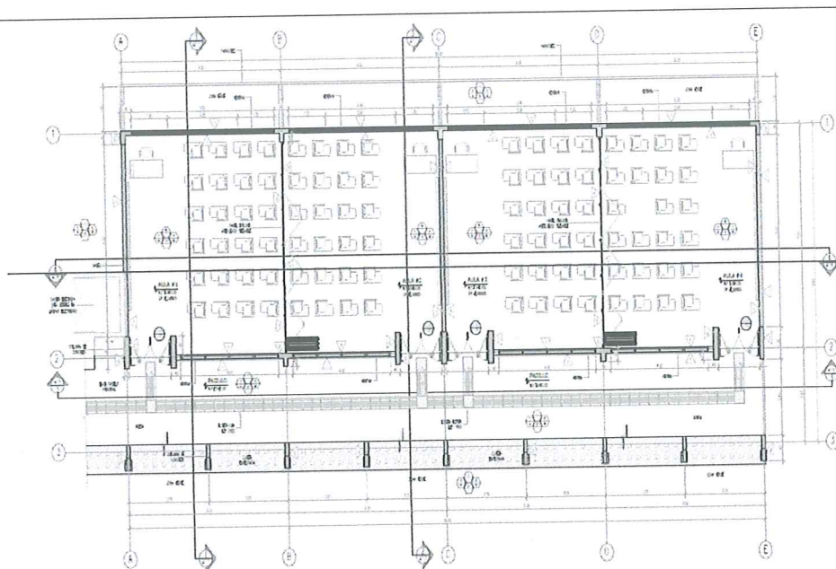
Planta de distribución del aula a construir
